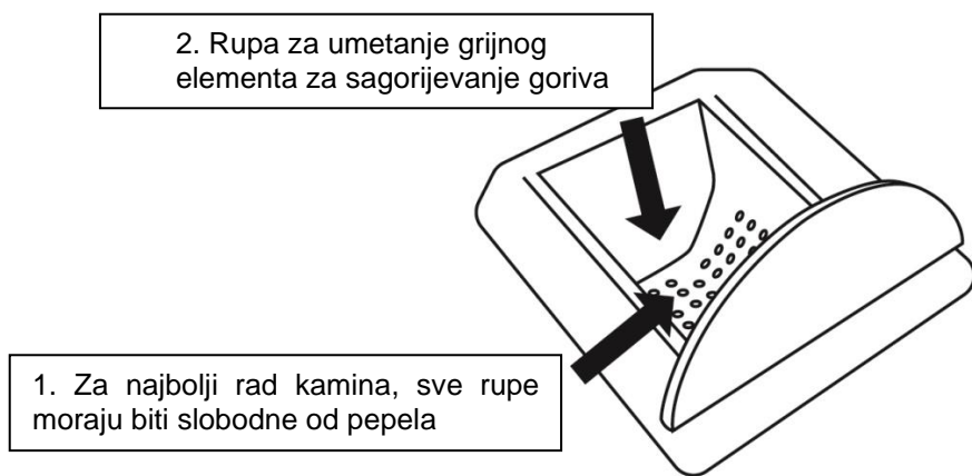
Slika 16. Gorionik
