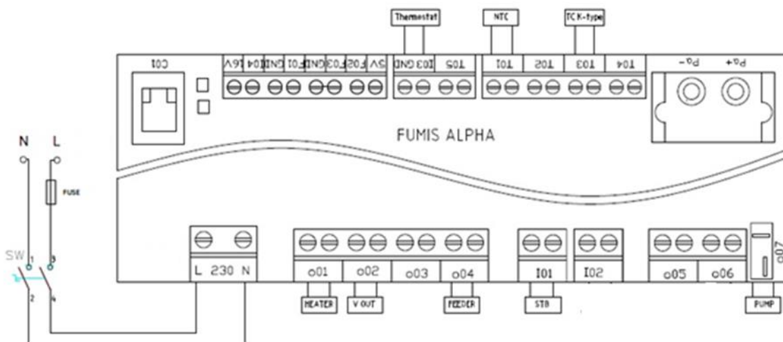
Slika 30: Elektro Šema
