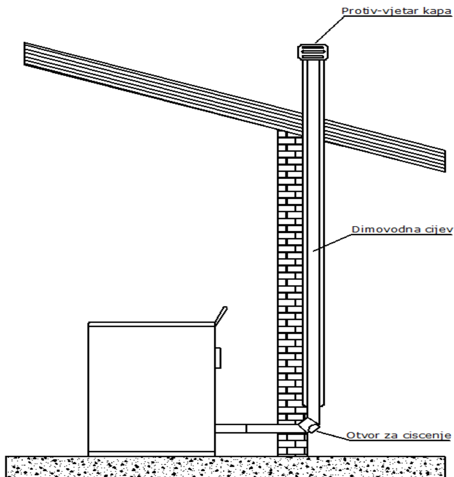
Slika 2: Dimnjak za kotao
