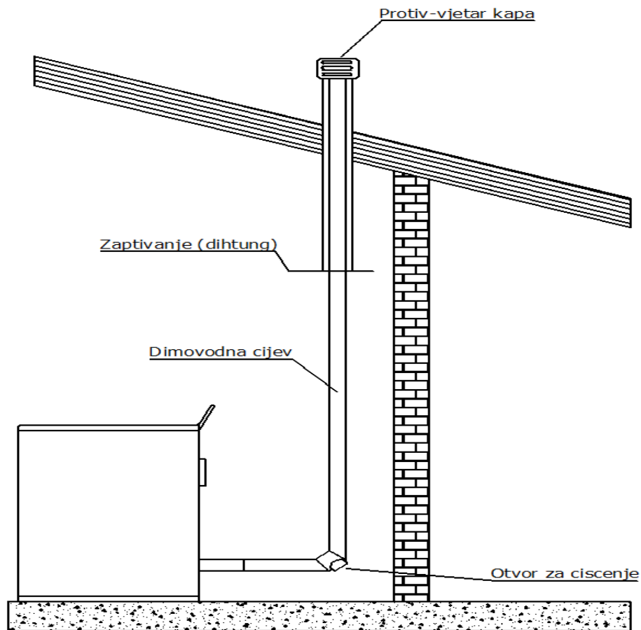
Slika 3: Izgled dimnjaka
