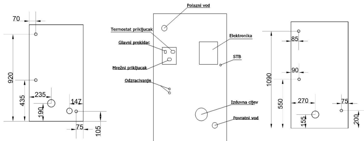
Slika 1. Poleđina kotla 15-lijevo; 23-desno
