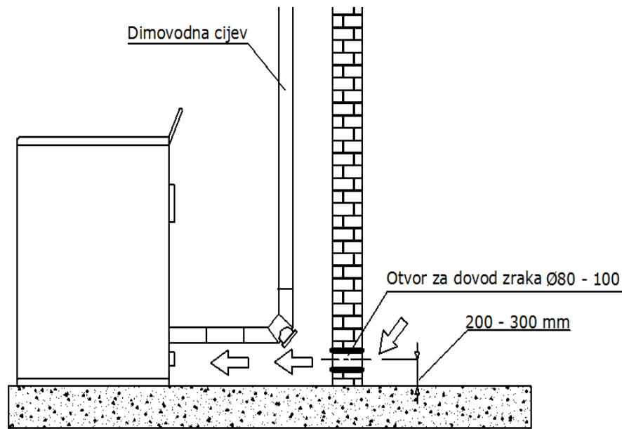
Slika 10. Minimalan prostor za postavljenje ventilacione rešetke
